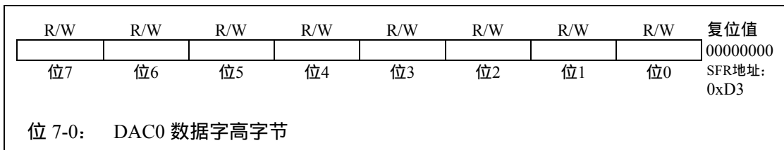
图 8.2 DAC0H: DAC0 高字节寄存器
