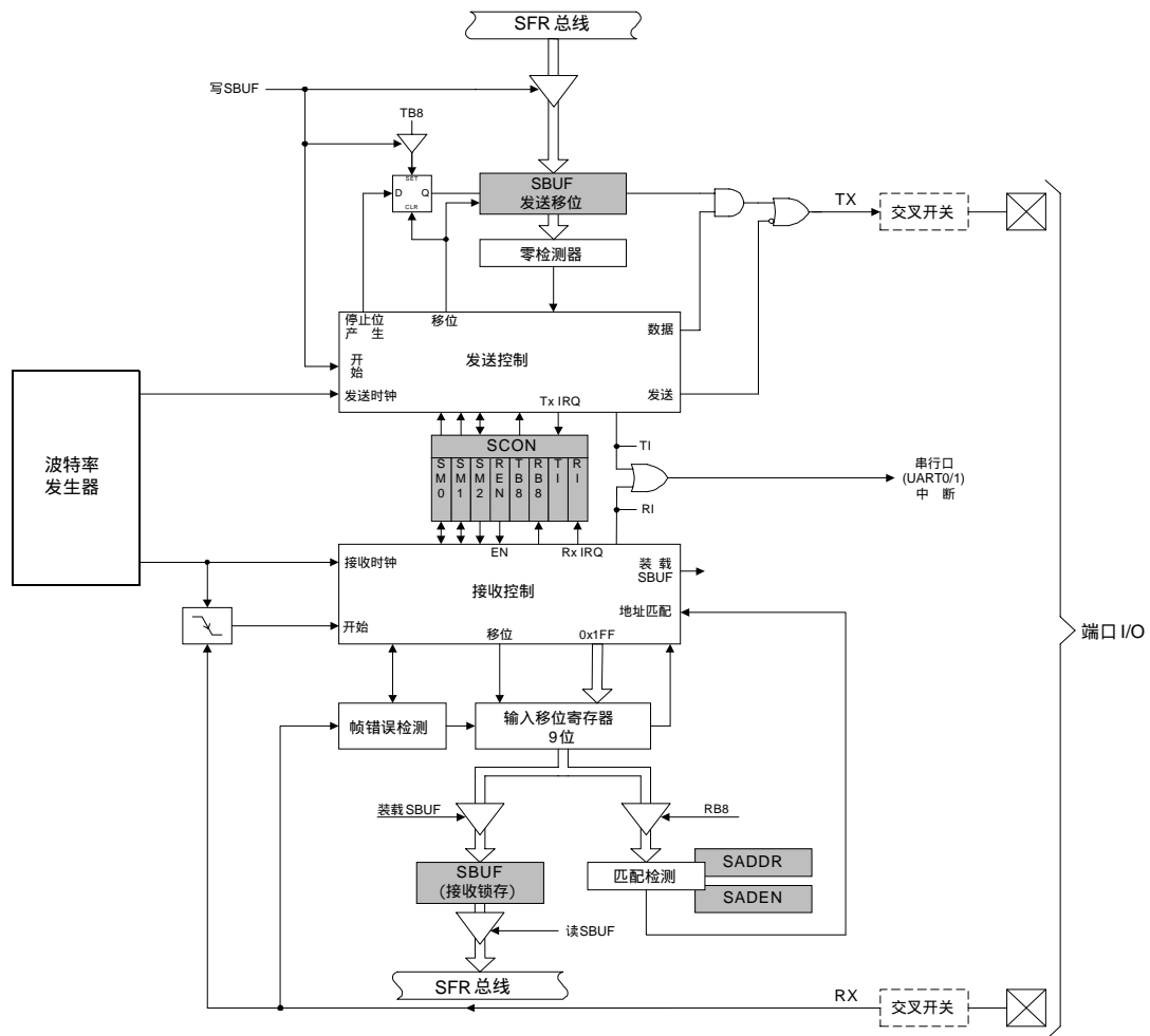
图 21.1 UART1 原理框图
