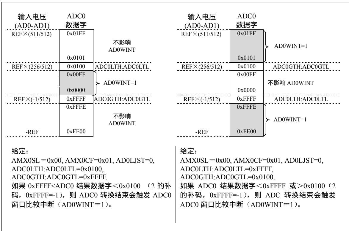
图 6.17 10 位 ADC0 窗口中断示例：右对齐的差分数据
