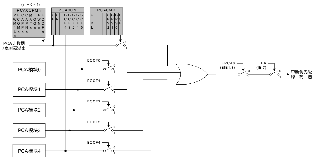
图 23.3 PCA 中断原理框图
