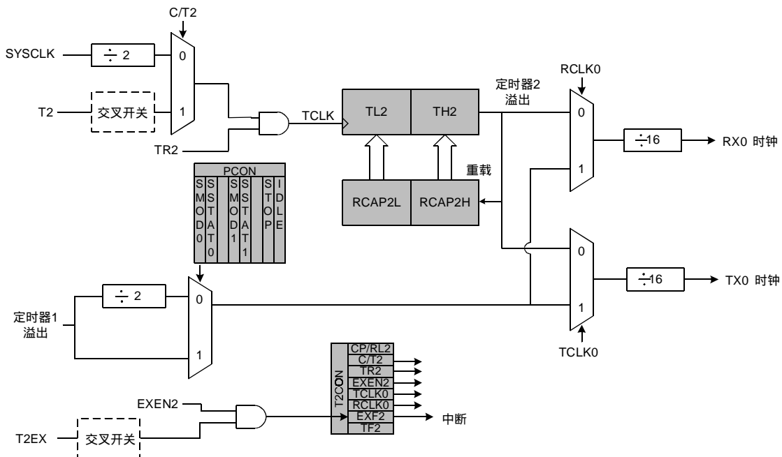
图 22.13 T2 方式 2 原理框图
