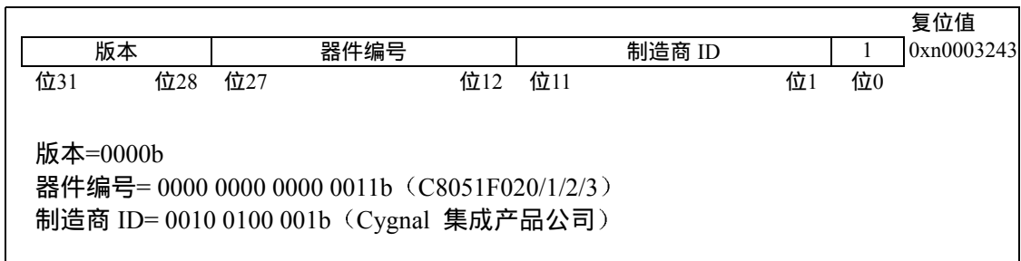
图 24.2 DEVICEID: JTAG 器件 ID 寄存器
