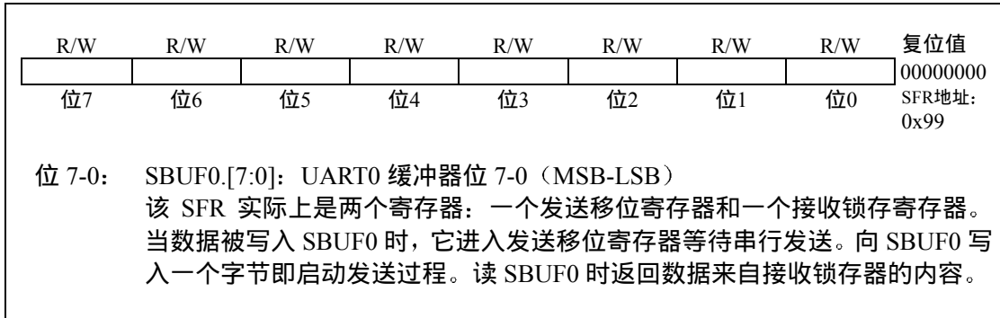
图 20.9 SBUF0: UART0 数据缓冲寄存器
