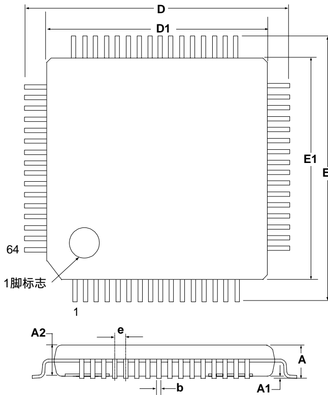
图 4.4 TQFP-64 封装图
