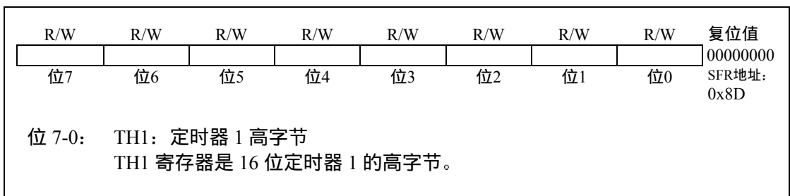
图 22.10 TH1: 定时器 1 高字节
