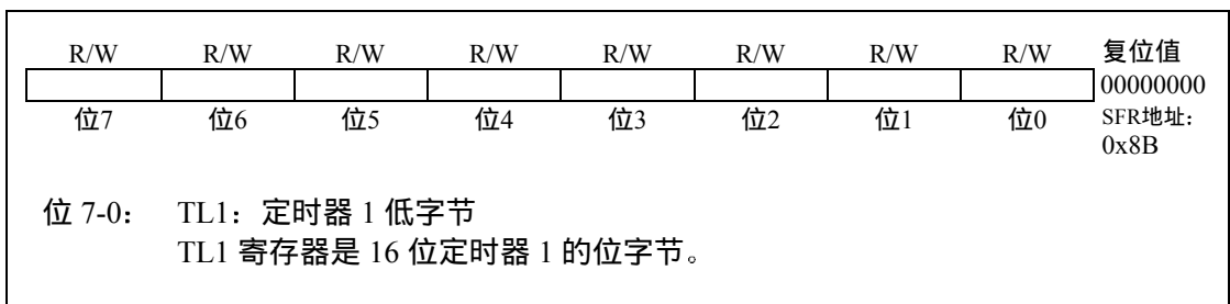
图 22.8 TL1: 定时器 1 低字节
