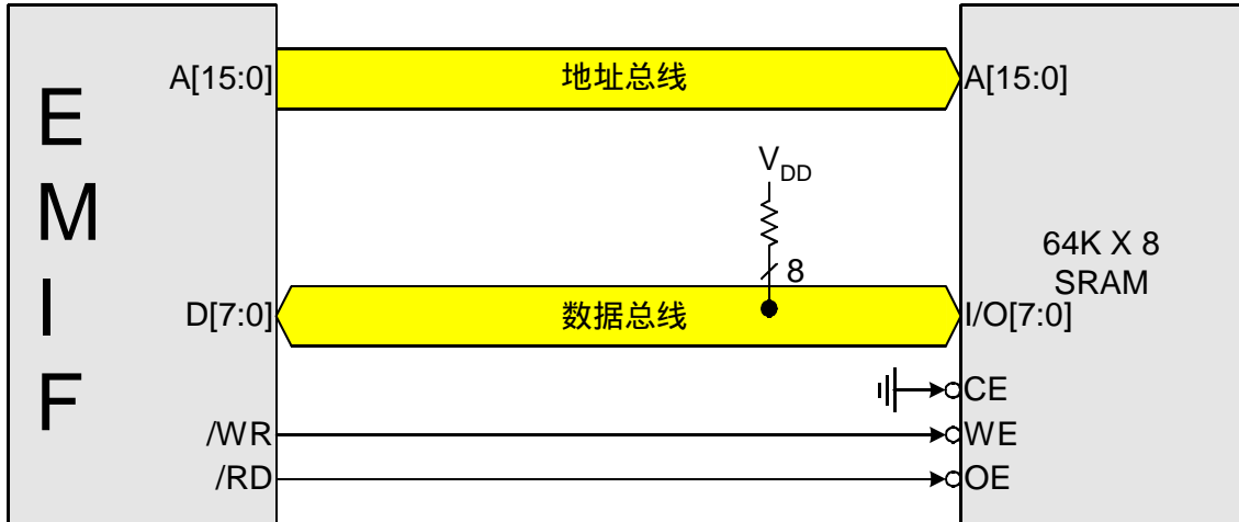
图 16.4 非复用方式配置示例
