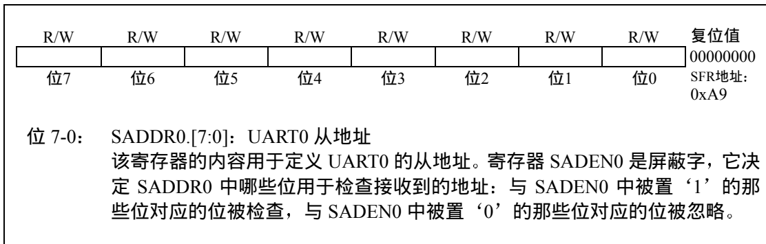
图 20.10 SADDR0: UART0 从地址寄存器
