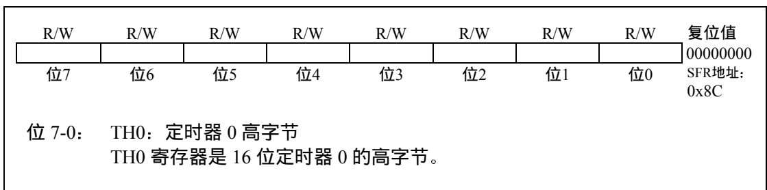
图 22.9 TH0: 定时器 0 高字节
