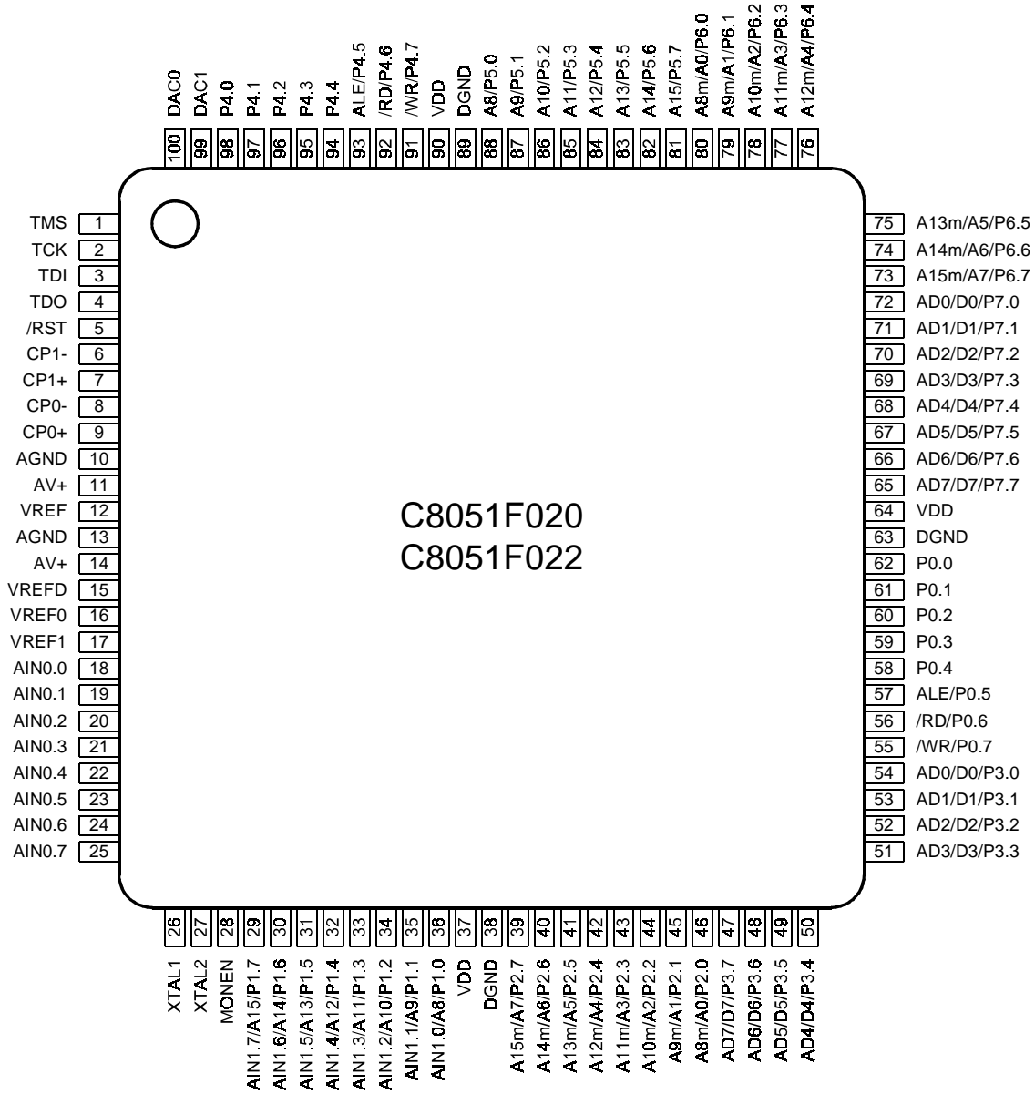
图 4.1 TQFP-100 引脚图
