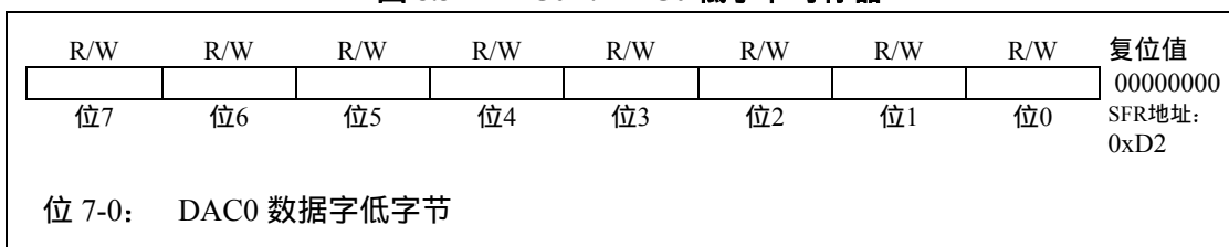
图 8.3 DAC0L: DAC0 低字节寄存器
