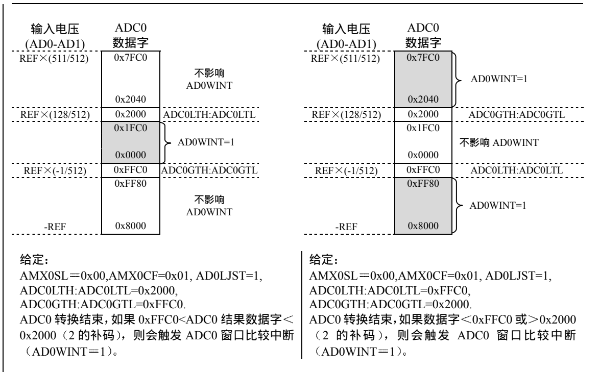
图 6.19 10 位 ADC0 窗口中断示例：左对齐的差分数据
