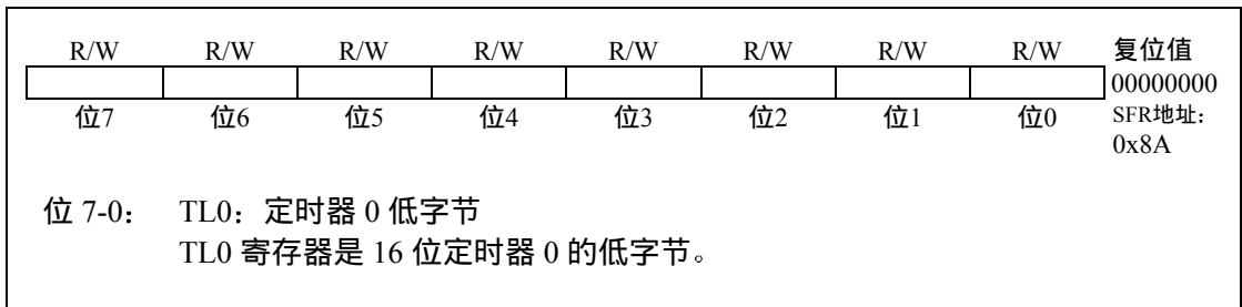
图 22.7 TL0: 定时器 0 低字节
