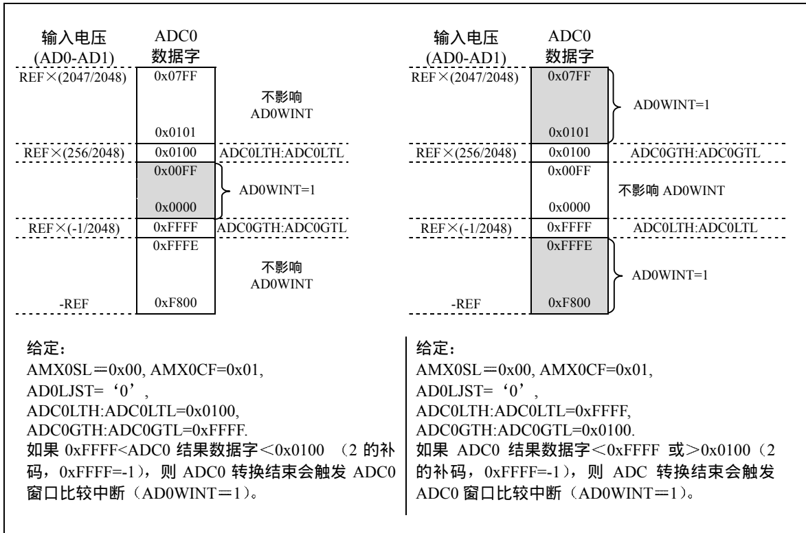
图 5.17 12 位 ADC0 窗口中断示例：右对齐的差分数据
