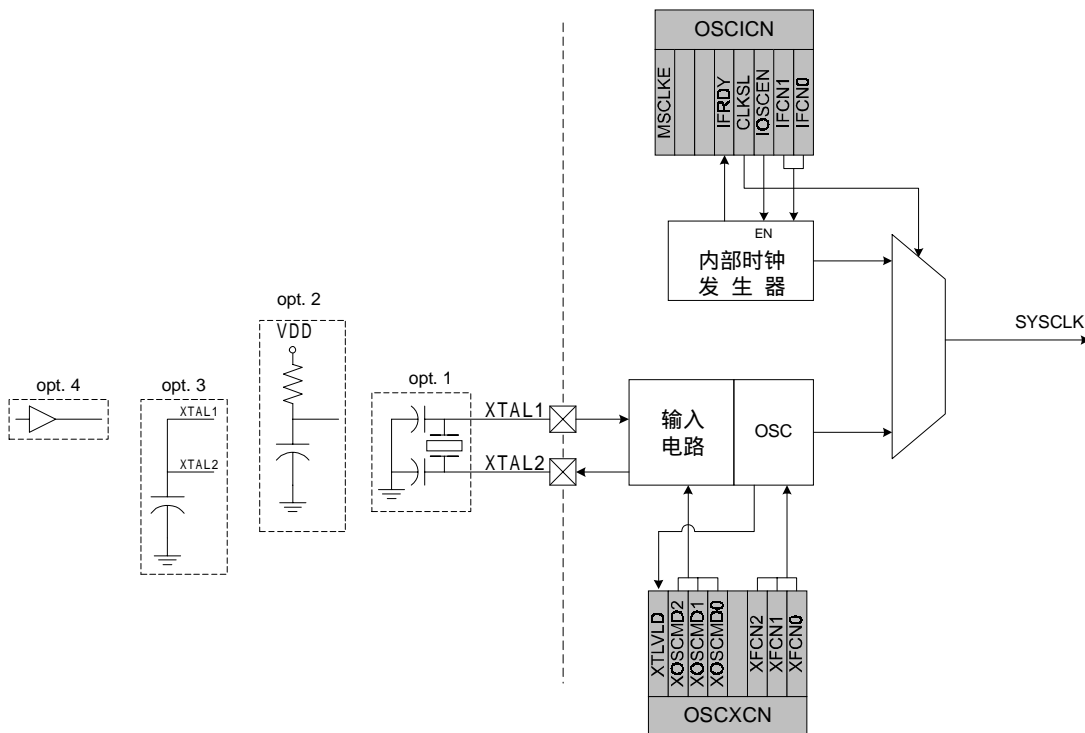
图 14.1 振荡器框图
