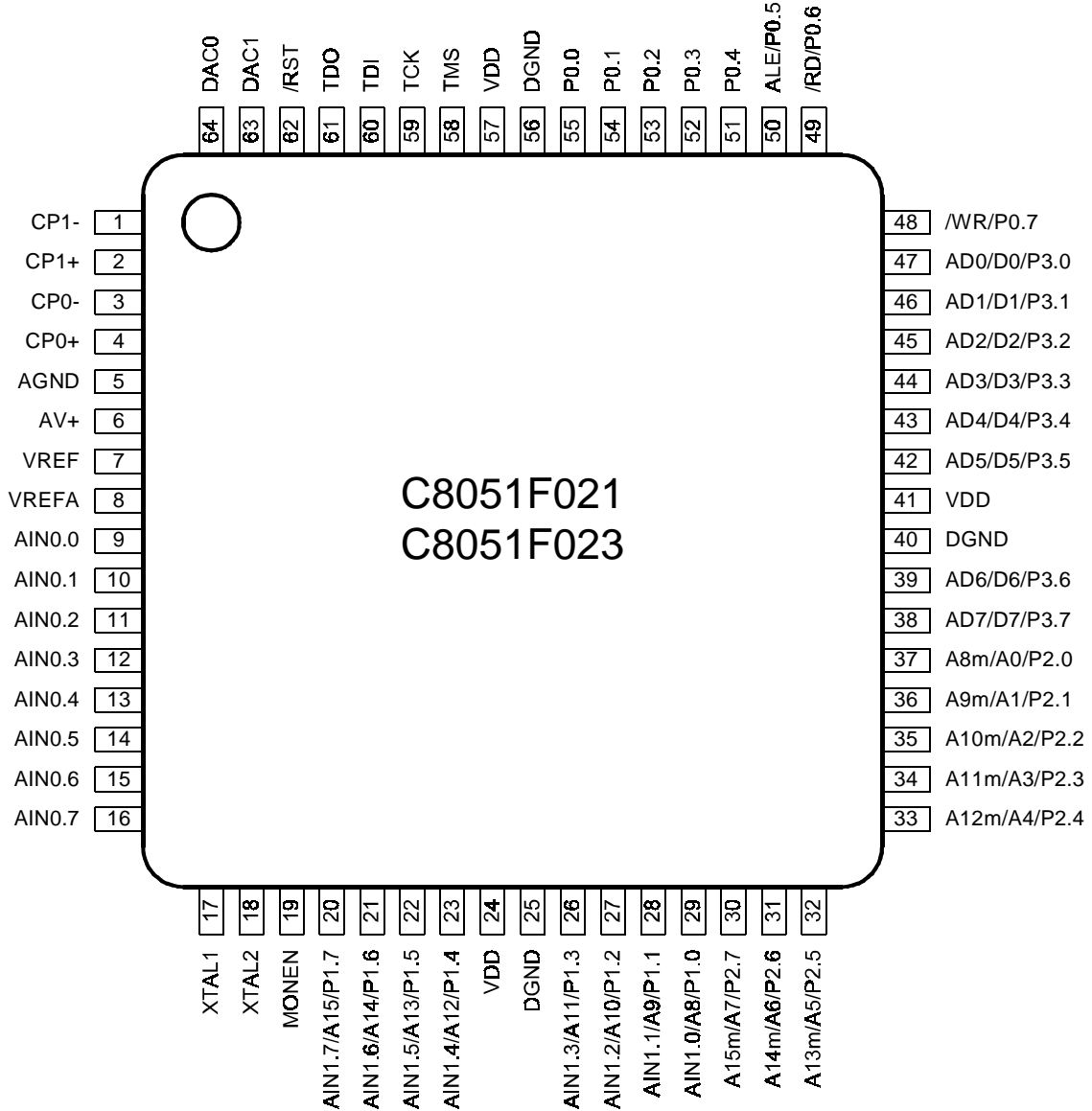
图 4.3 TQFP-64 引脚图
