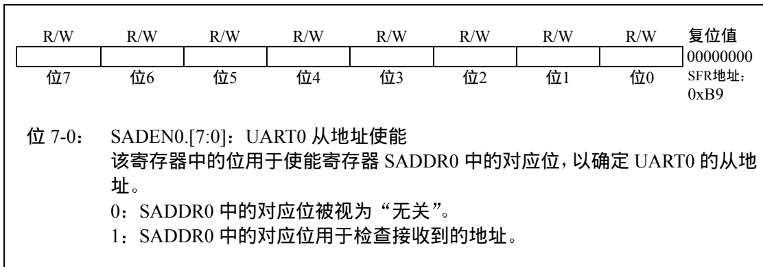
图 20.11 SADEN0: UART0 从地址使能寄存器
