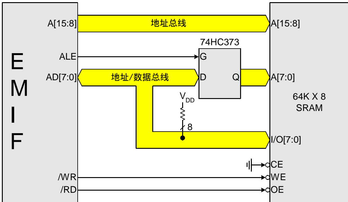
图 16.3 复用方式配置示例
