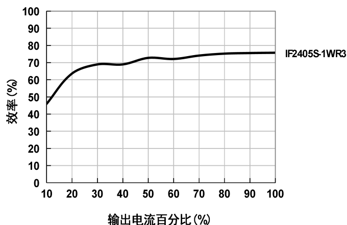
效率Vs输出负载 (Vin=24V)
