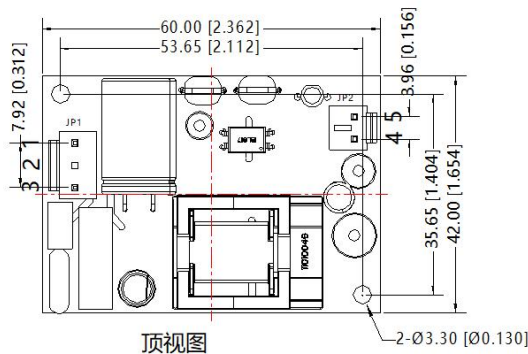
顶视图
